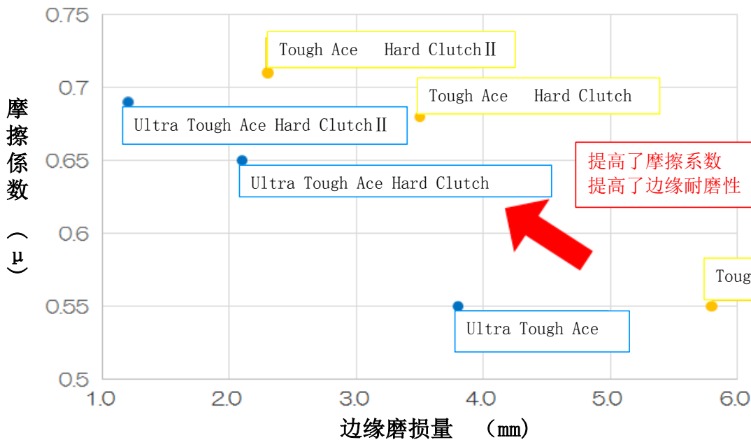
摩擦系数 (dry) 与边缘磨损量
